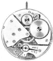
12''' cal. 1120
